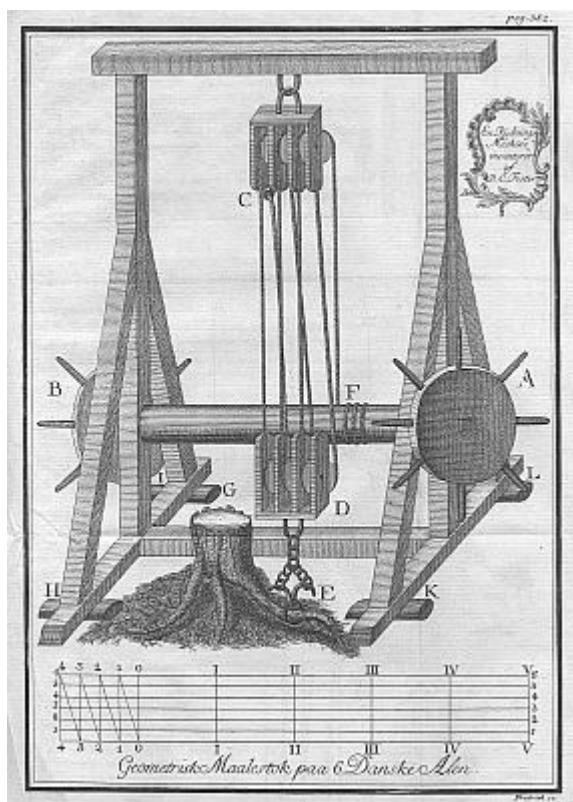
Illustration til Fester's »Forslag til en Rydnings-Maskine«.
